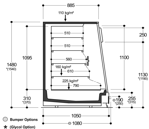
Sezione GranVadaj 15 L
