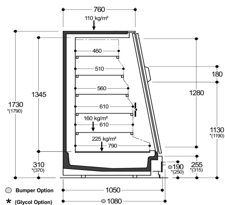
Sezione GranValdj sliding 17_L
