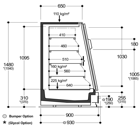
Sezione GranValdj sliding 15_N
