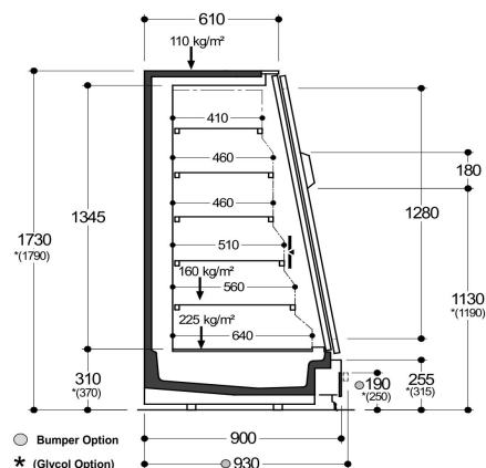
Sezione GranValdj sliding 17_N
