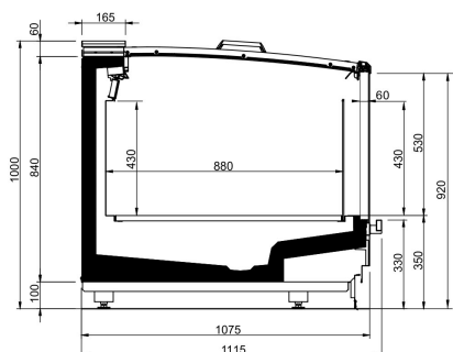
Sezione GranDrake_Linear_Sliding Covers
