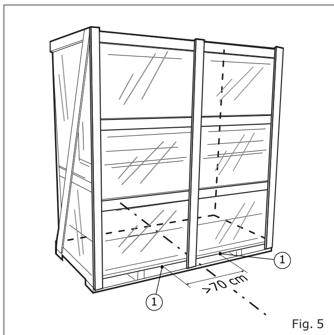
1. Løftepunkter
