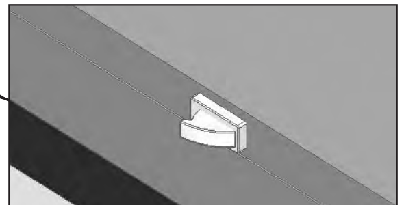
Microinterrupteur du ventilateur intérieur (avec la porte ouverte: ventilateur deconnecté)
