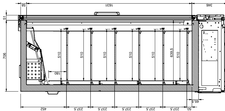
A-A 1:10
