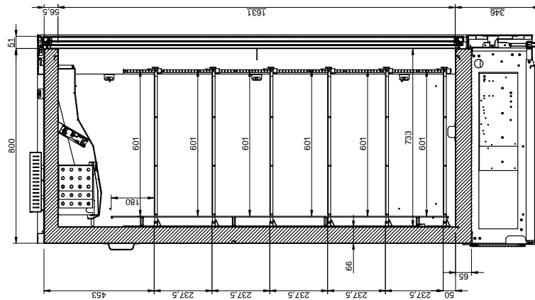
B-B 1:10
