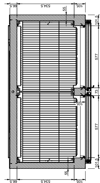
B-B 1:10
